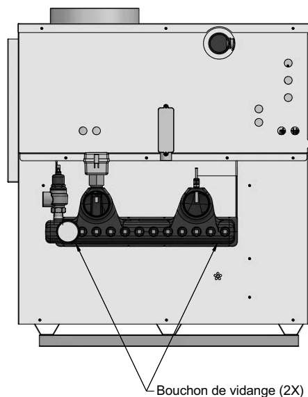
Figure 1-2B Égoutter les unit_Models 1000 - 2100
