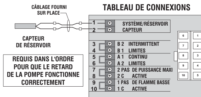
Figure 5-8_Capteur à distance pour retard de pompe
