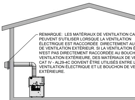
VENTILATION LATÉRALE/ÉLECTRIQUE
