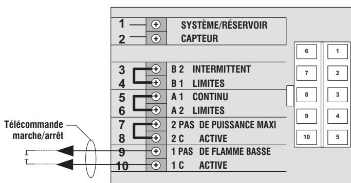
Figure 5-5_Télécommande marche/arrêt Chaudière ou chauffe-eau
