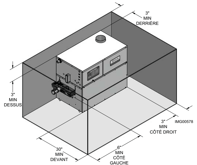
Figure1-1 _Espaces intérieurs d'une construction combustible
