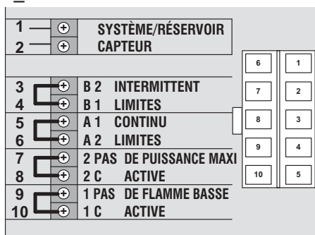
Figure 5-5_Télécommande marche/arrêt Chaudière ou chauffe-eau
