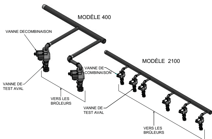
Figure 3-2_Schéma d'un circuit de gaz de Chauffe-eau classique
