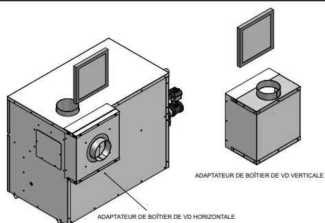
Figure 2-10 Fixation de l'adaptateur de boîtier DV à l'appareil
